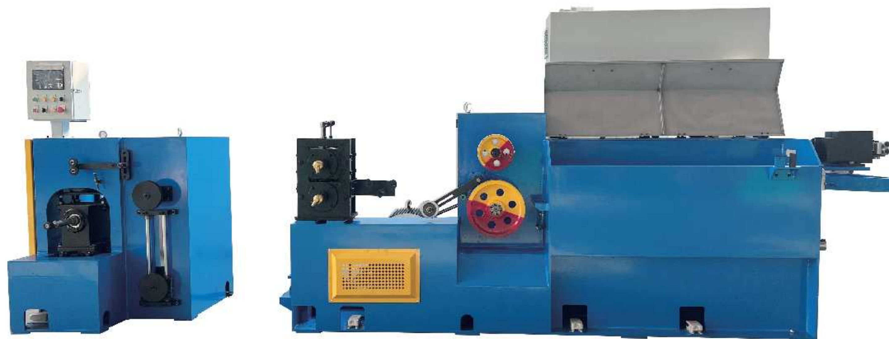
进线 \phi 2.4 出线 \phi 0.9 Inlet wire \phi 2.4 Outlet wire \phi 0.9
